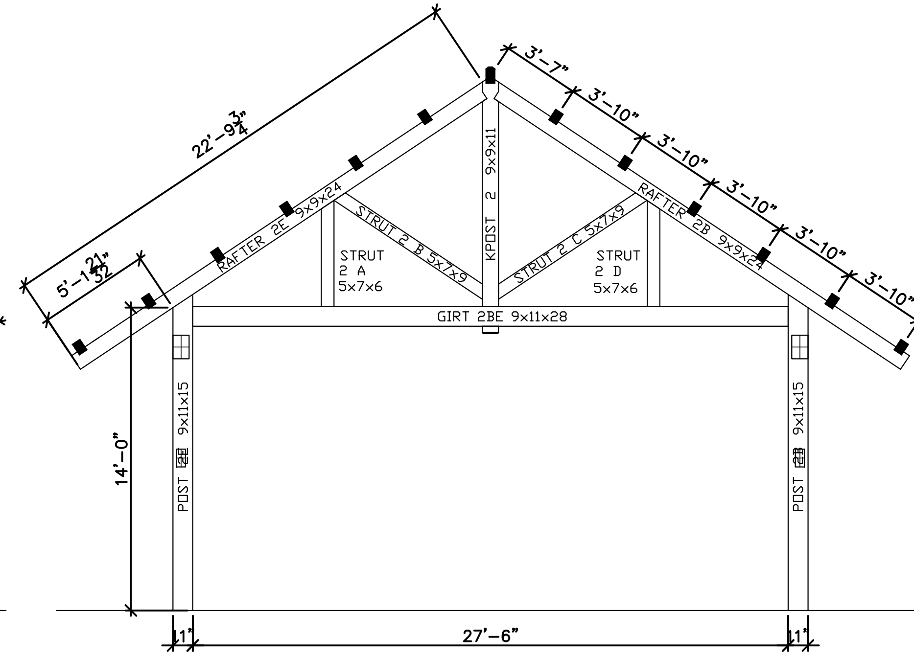
BENT 2
