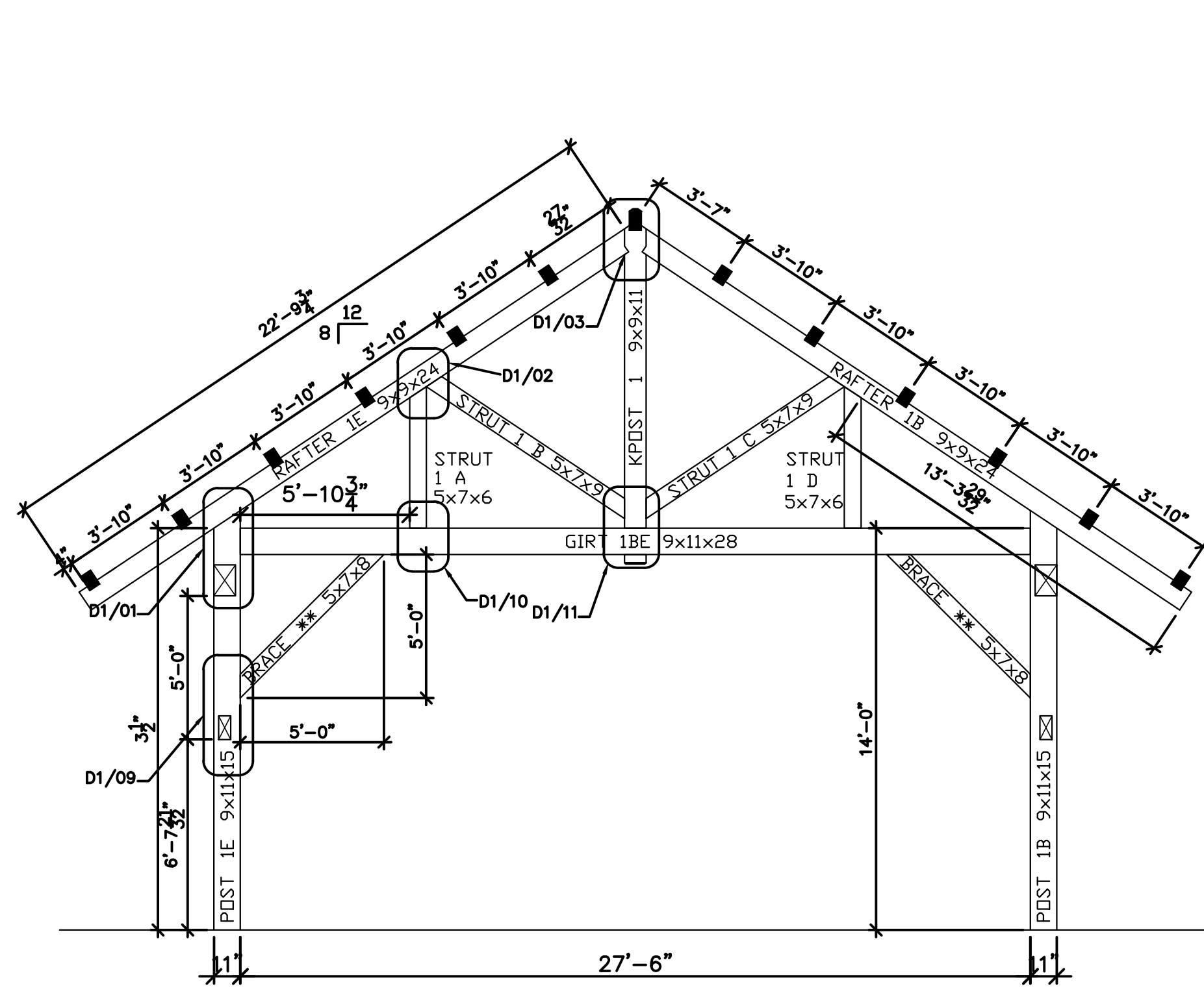
BENT 1
