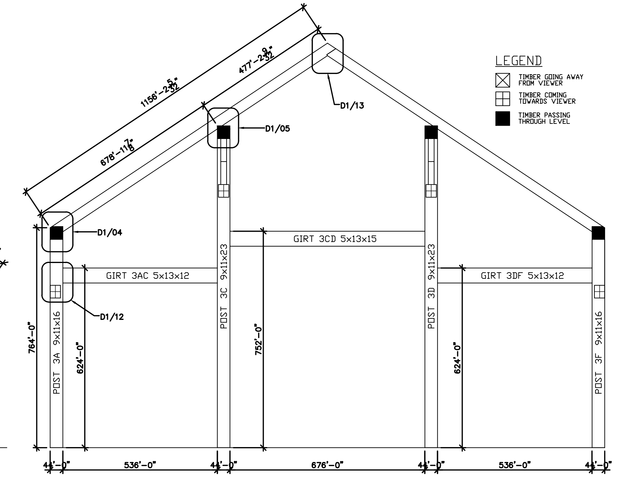
BENT 3
