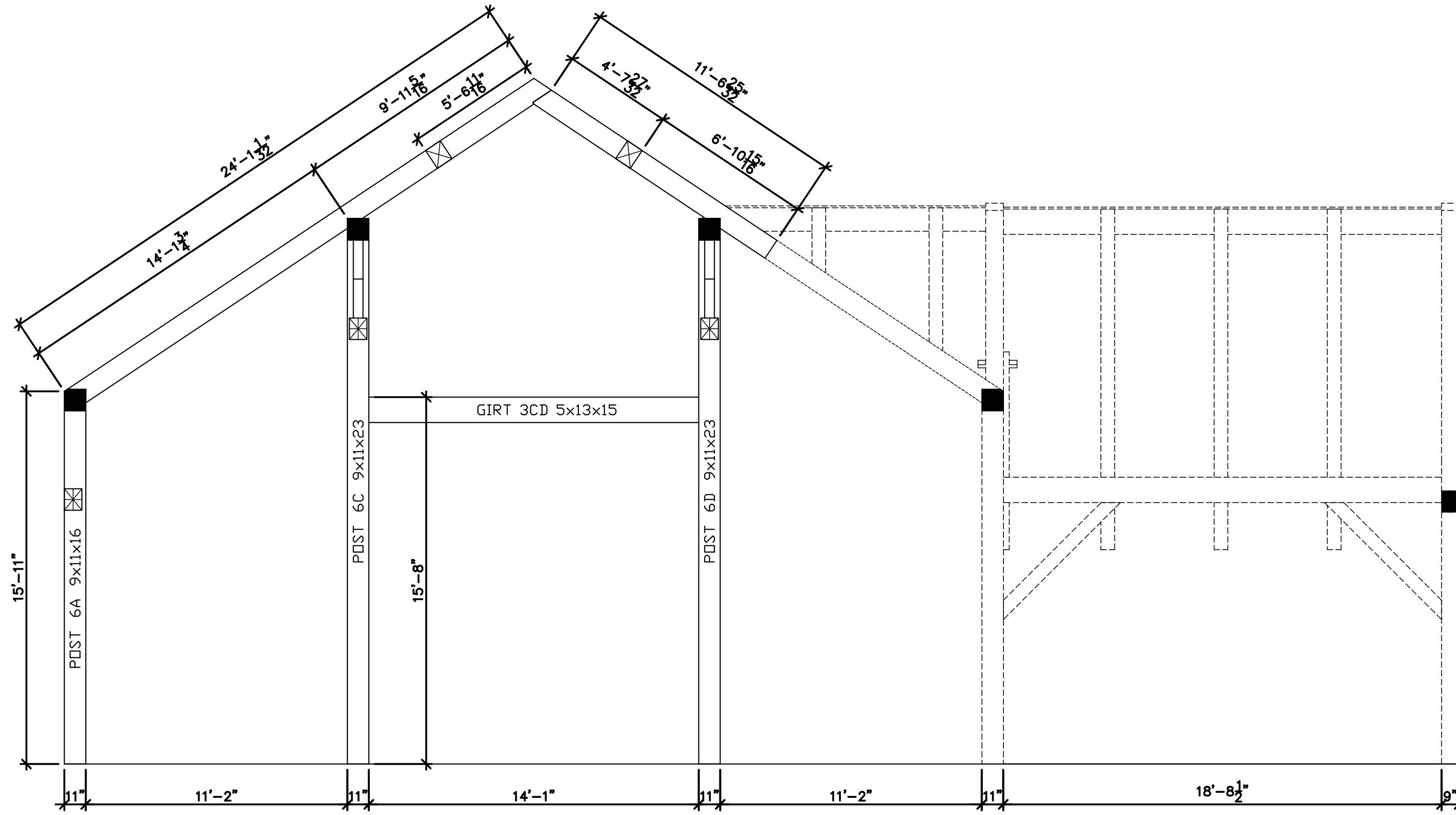
BENT 6
