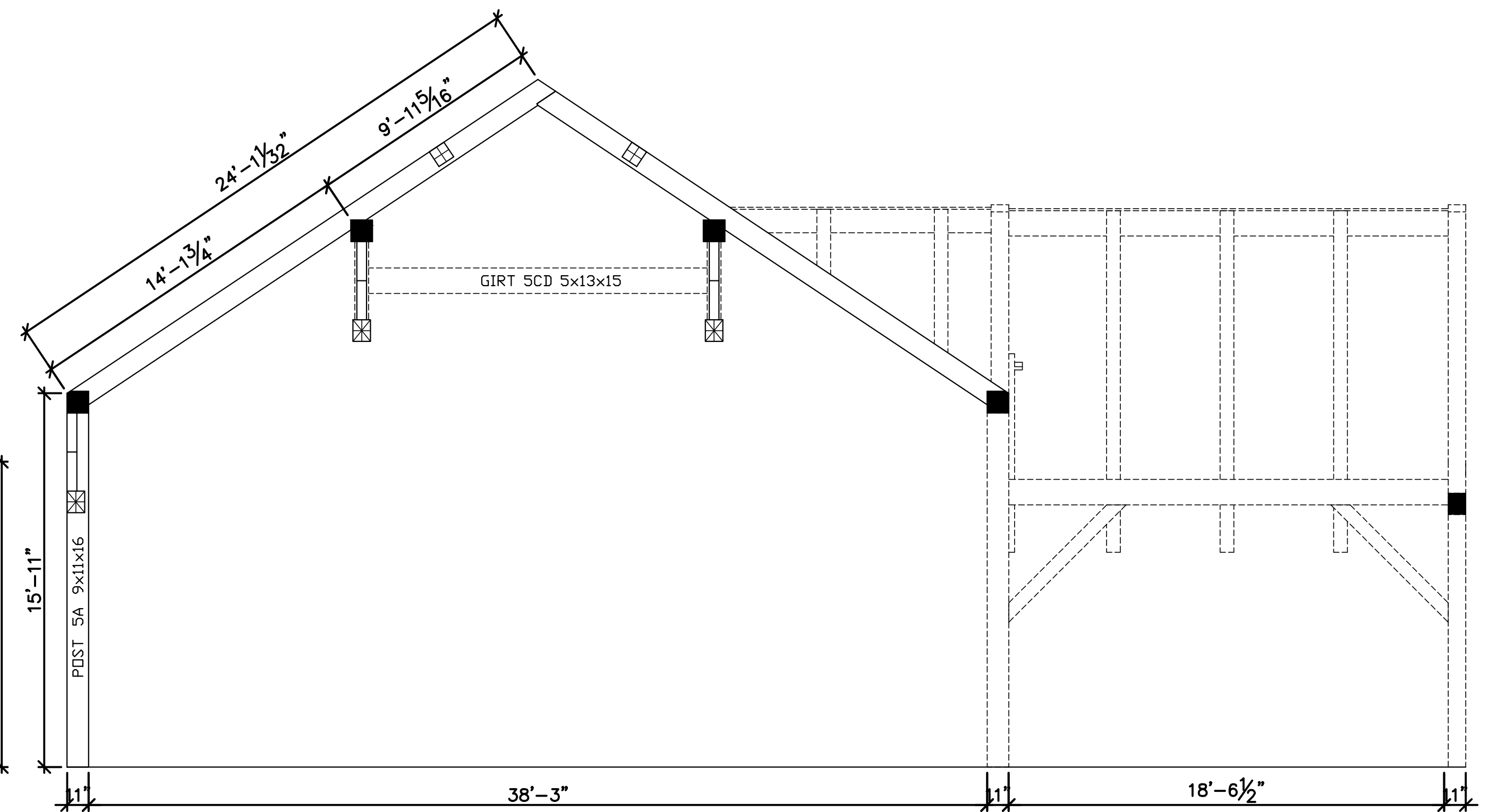
BENT 5
