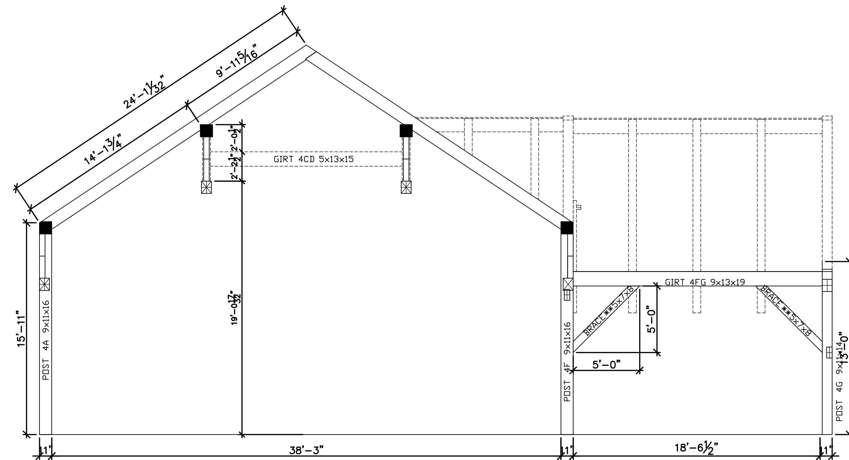
BENT 4
